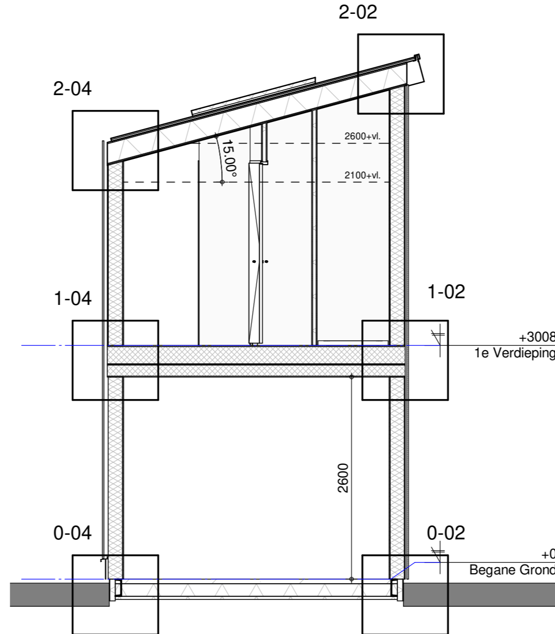
Doorsnede
