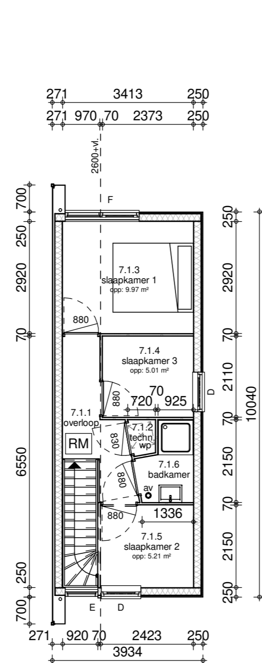
1e Verdieping
