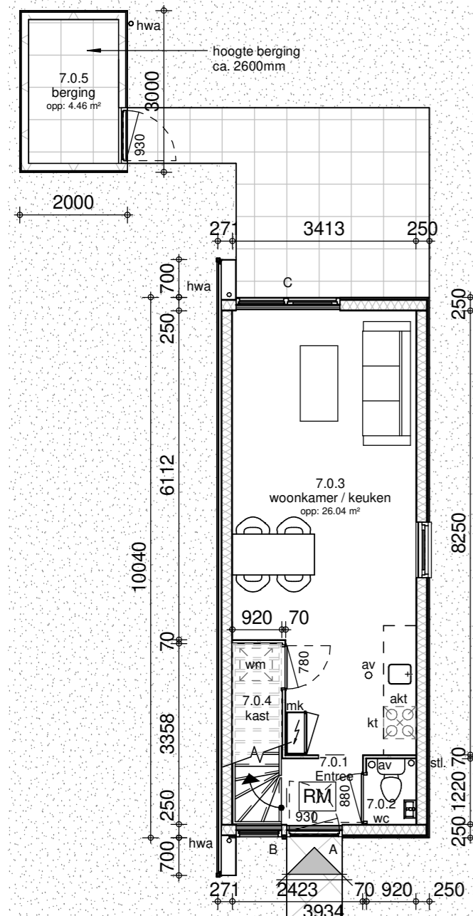
Begane Grond
